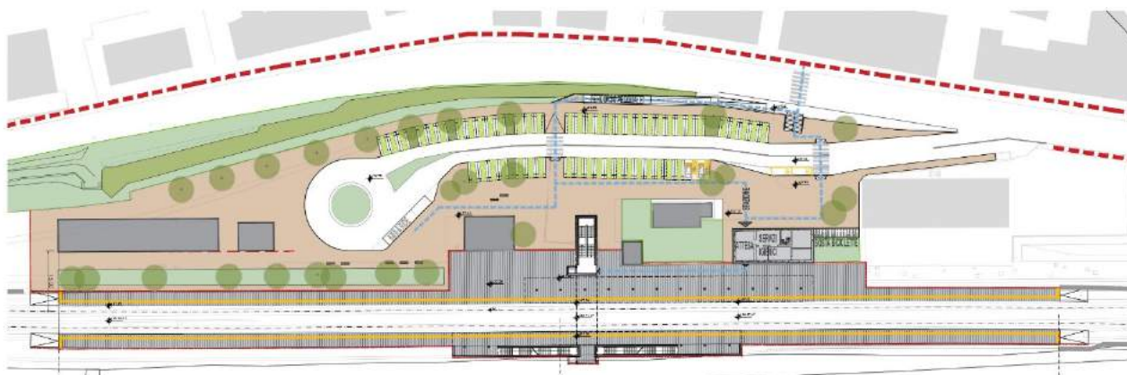
Figura 21 Pianta stazione Serra San Quirico
